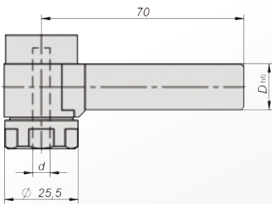
CoolSpeed mini 90 D = Ø16 mm 700500016
